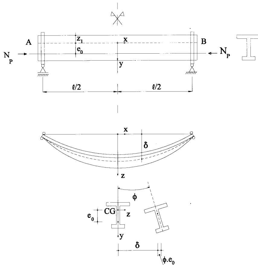
Figura 2.3 - Viga protendida de seção duplo T. [ CATANIA & COCCHI (1985) ]
