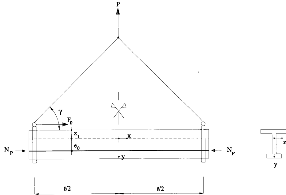
Figura 3.15 - Viga protendida em suspensão. [ CATANIA & COCCHI (1985) ]
