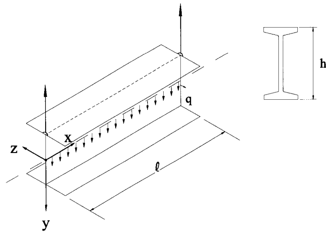
Figura 3.20 - Viga de seção duplo T simétrico suspensa por cabos verticais.
