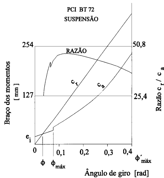
Figura 4.6 - Viga fissurada para \phi > \phi_{m\acute{a}x} [ MAST (1993) ]
