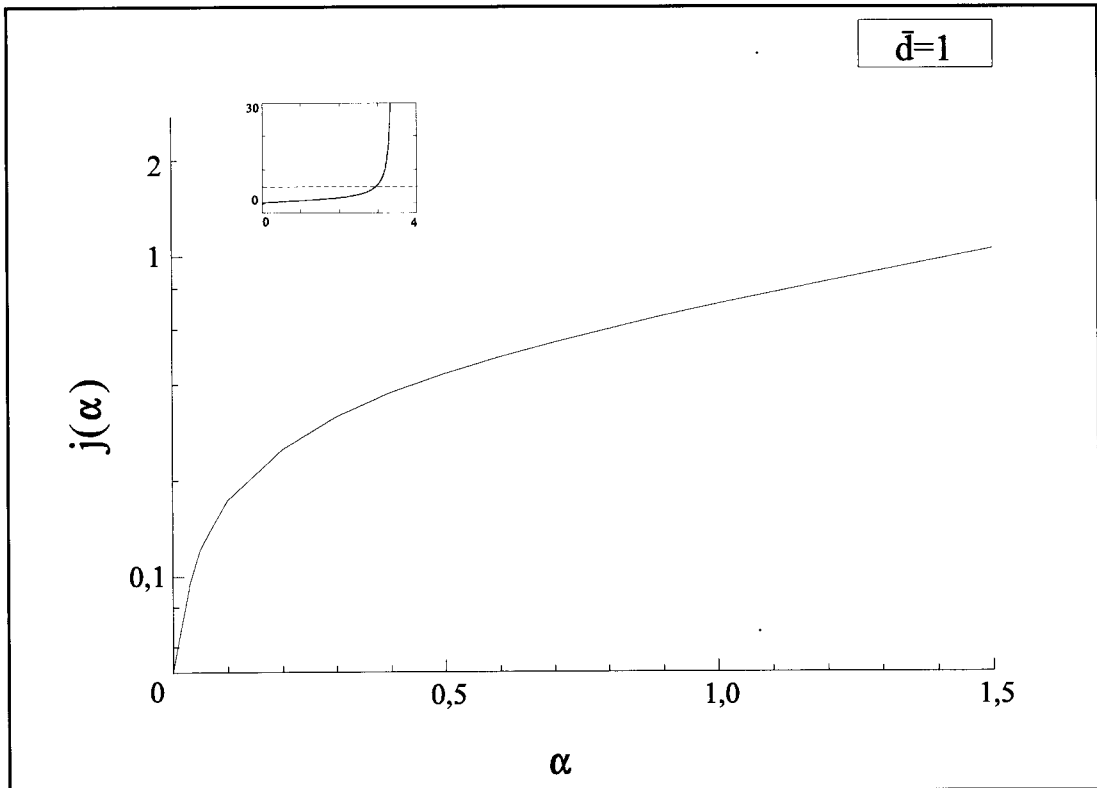
Figura 3.5 - Gráfico da função j(\alpha) para \bar{d}=1 .
