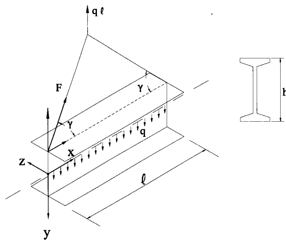
Figura 3.21 - Viga de seção duplo T simétrico suspensa por cabos inclinados.
