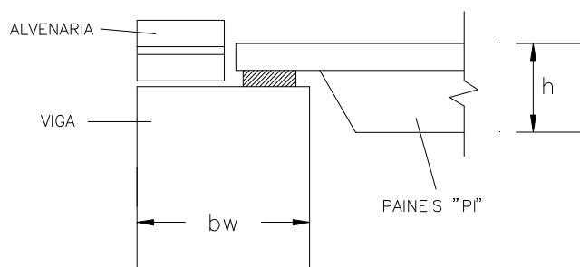
FIGURA 31 - Detalhe de Ligação Viga-Laje de Extremidade
