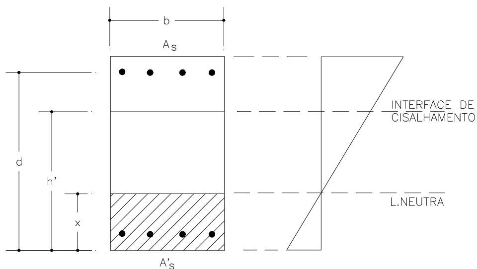
FIGURA 60 – Situação da Linha Neutra em Relação à Interface de Cisalhamento
