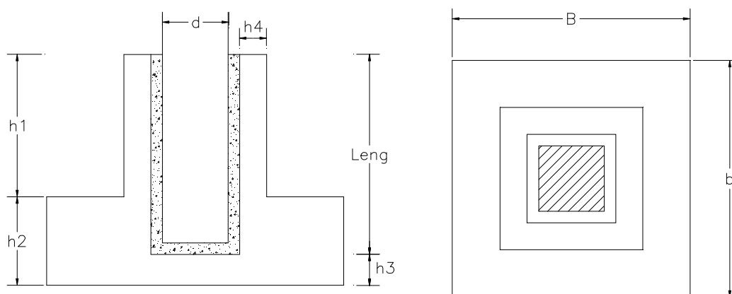
FIGURA 66 – Cálice de Fundação
