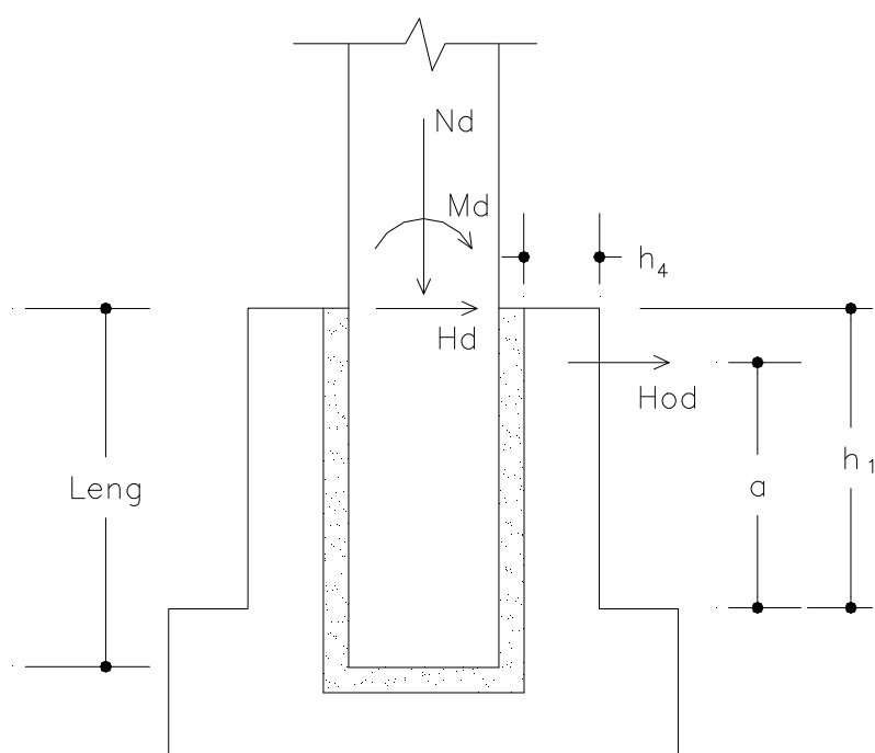
FIGURA 68 – Esquema das Ações Solicitantes no Cálice
