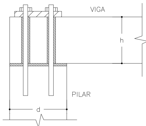
FIGURA 27 – Ligação Rígida Pilar-Viga de Topo
