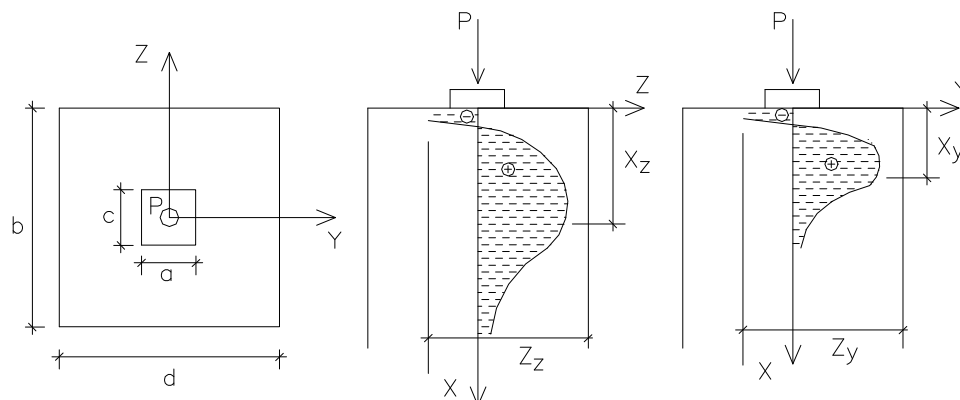
FIGURA 26 - Distribuição das Tensões de Fendilhamento ao Longo do Elemento Carregado (LEONHARDT & MONNIG)
