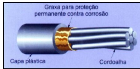
Figura 4.7 - Cordoalha engraxada (CAUDURO, 1997)
