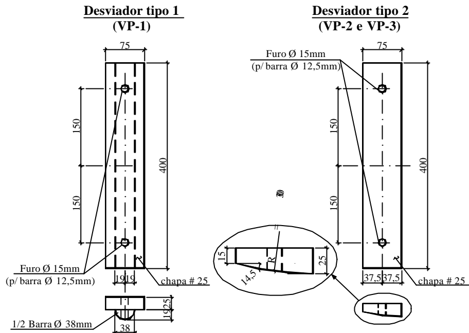
Figura 4.10 - Detalhe dos desviadores
