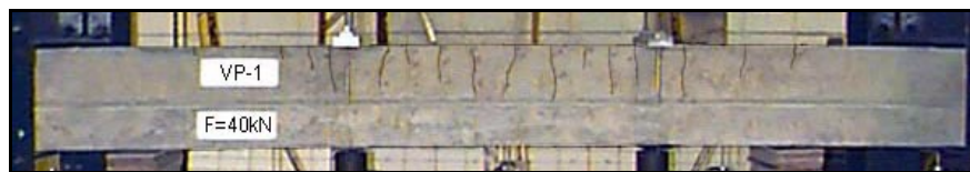
Fim da primeira etapa, com F = 40\text{kN} .
