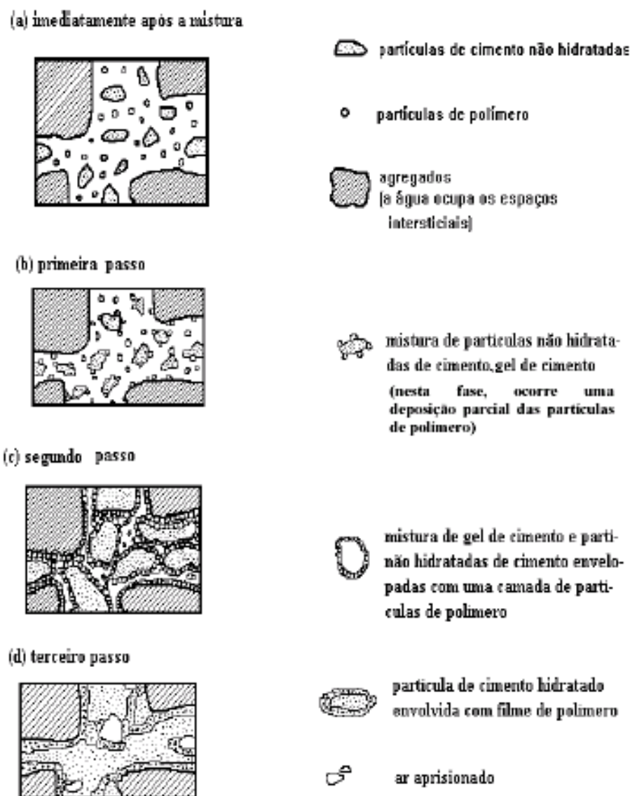
Figura 2.2 – Modelo idealizado de formação do concreto de cimento polímero (OHAMA, 1998 apud. PERUZZI, 2002)
