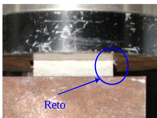
Figura 4.51 – Almofada do compósito
