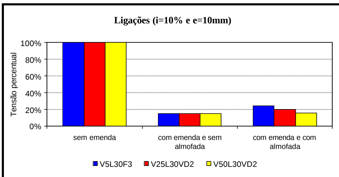
Figura 4.63 – Relação entre as tensões ( i = 10\% e e = 10\text{mm} ) – Série 2
