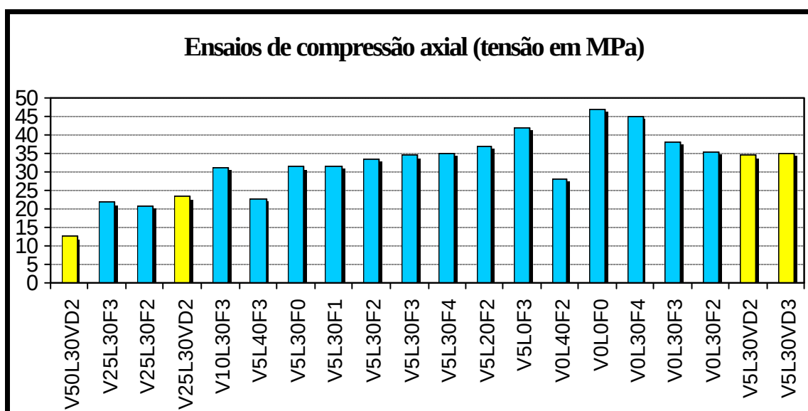
Figura 4.1 – Gráfico comparativo das tensões para ensaio de compressão axial
