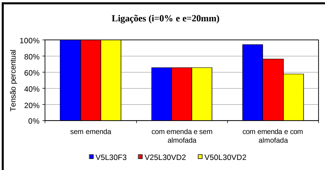
Figura 4.65 – Relação entre as tensões ( i = 0\% e e = 20\text{mm} ) – Série 4
