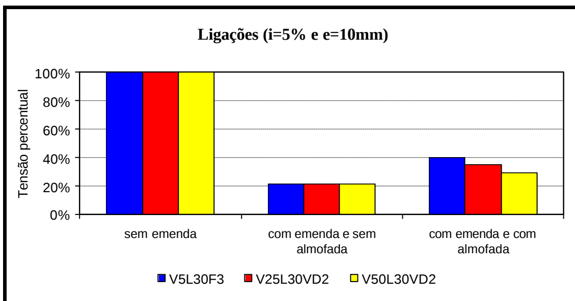
Figura 4.66 – Relação entre as tensões ( i = 5\% e e = 10\text{mm} ) – Série 5
