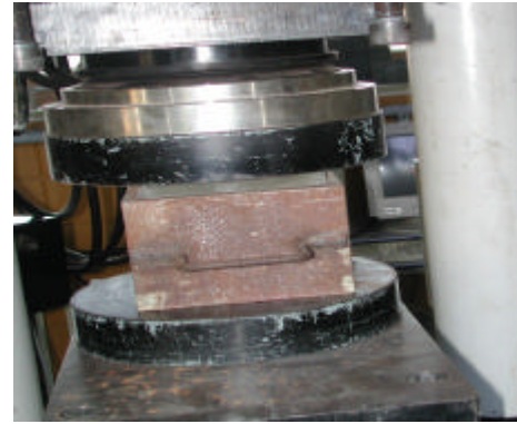
Figura 3.19c – Aplicação de carga em placa de 15cm x 15cm
