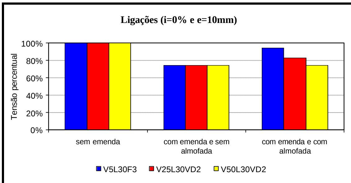
Figura 4.62 – Relação entre as tensões ( i = 0\% e e = 10\text{mm} ) – Série 1
