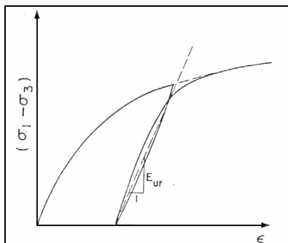
Figura 3.4 – Diagrama tensão-deformação da relação de carregamento e descarregamento, BOULANGER et al (1993).
