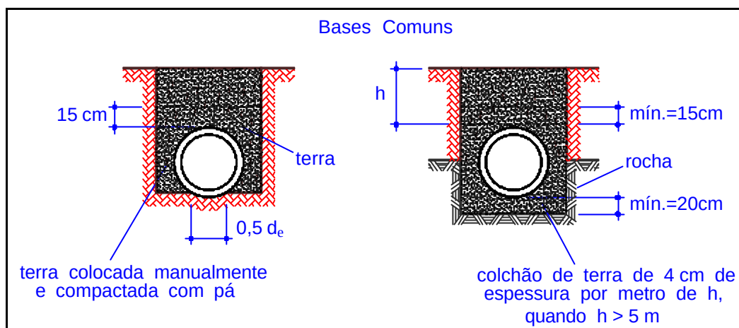
Figura 2.11 – Bases comuns ou Classe C (instalação em vala), adaptado por EL DEBS (2003).
