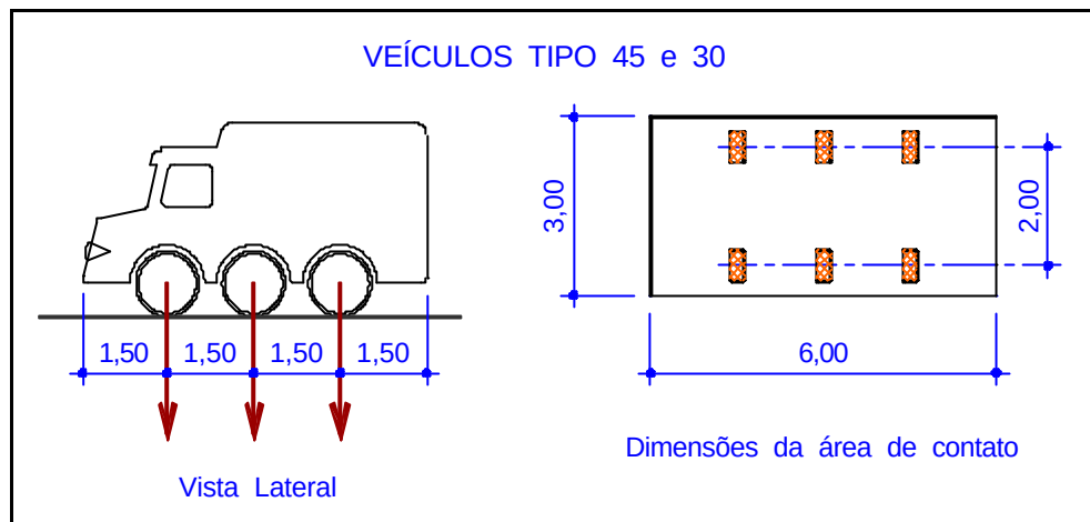
Figura 5.24 – Características do veículo-tipo
