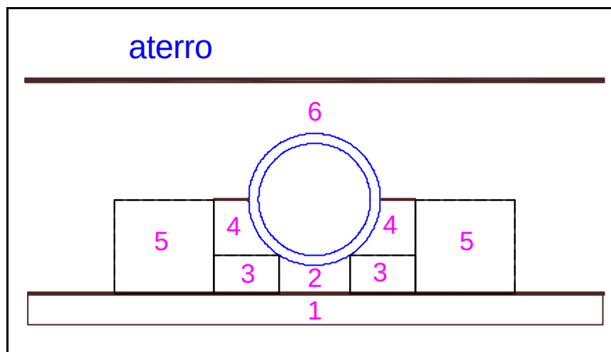
Figura 4.5 – Distribuição dos solos – SIDD.
