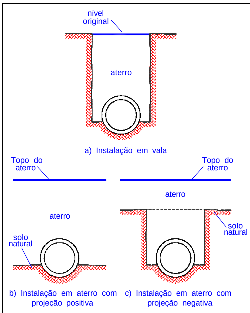
Figura 2.8 – Tipos básicos de instalação.
