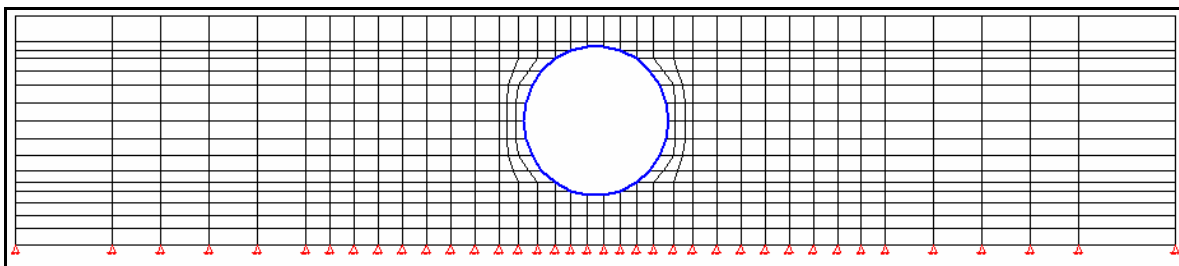
Figura 4.2 – Malha usada no trabalho.
