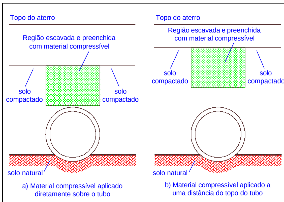
Figura 2.9 – Instalação em vala induzida, EL DEBS (2003).
