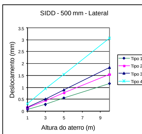
Figura 5.2 – Deslocamento horizontal nos flancos ( d_i = 500 mm)
