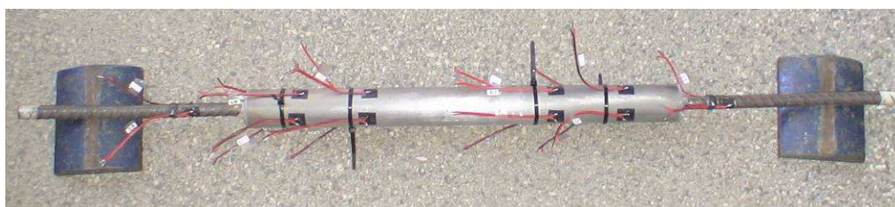
Figura 3.18 – Emenda com extensômetros
