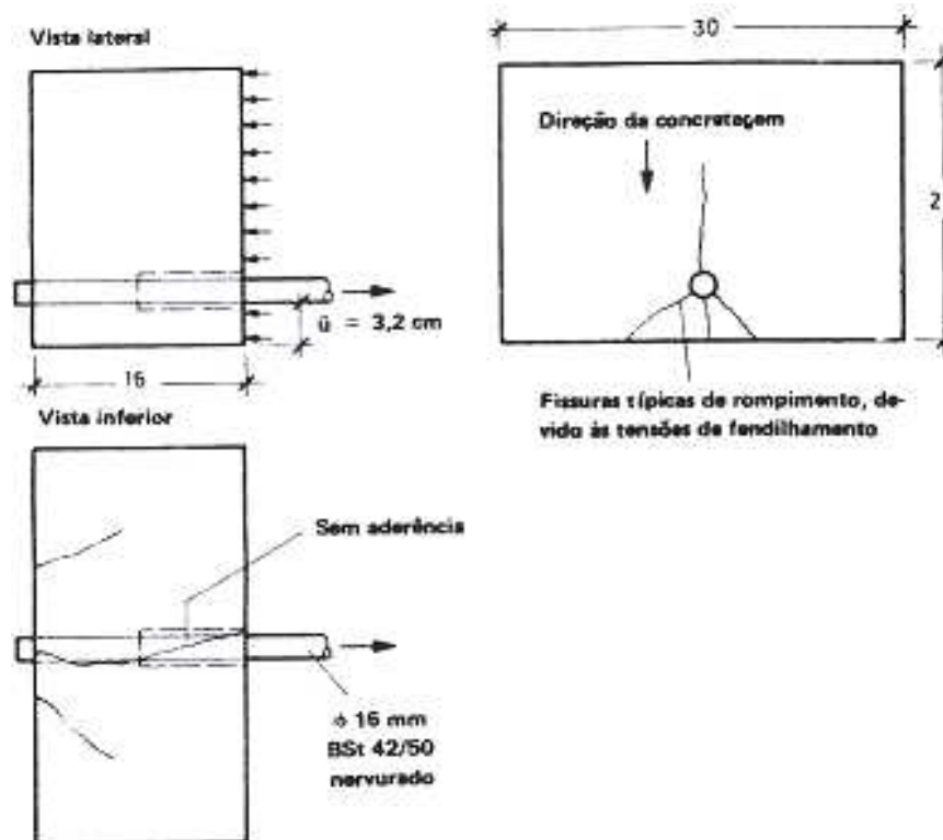
Figura 2.20 – Fissuras devido ao fendilhamento (Leonhardt, 1978)
