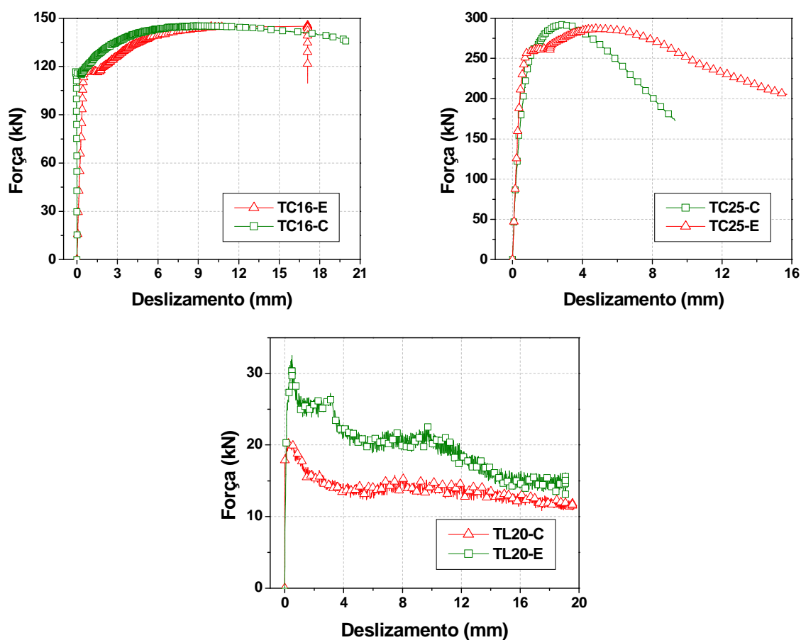
Figura 4.18 – Curva força-deslizamento das emendas TC16-C e TC16-E, TC25-C e TC25-E, e TL20-C e TL20-E
