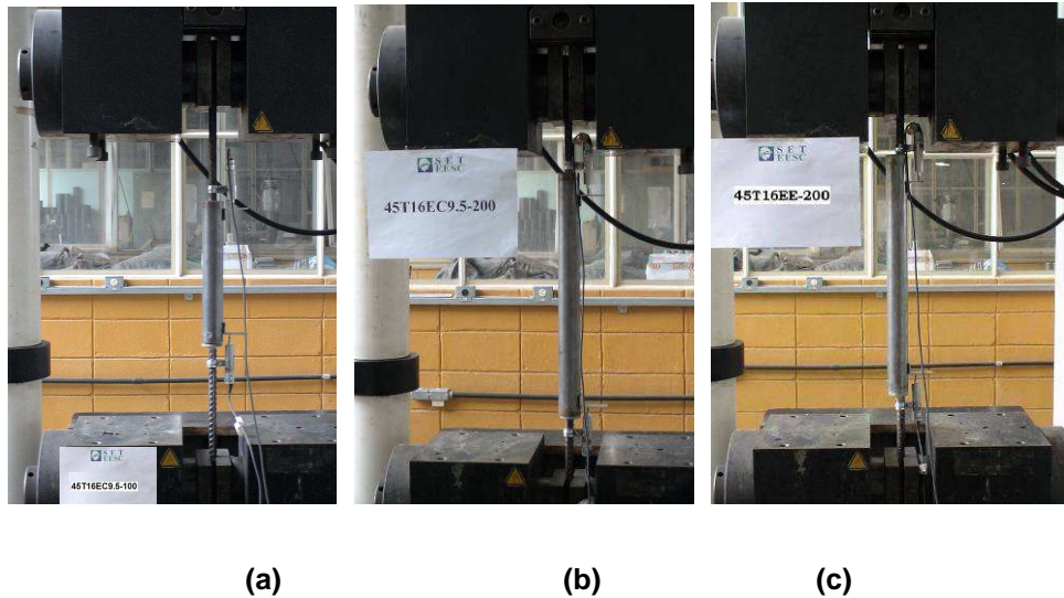
Figura 4.19 – Emendas sendo ensaiadas a) 45T16EC9.5-100, b) 45T16EC9.5-200 e c) 45T16EE-200
