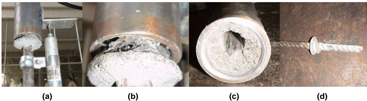
Figura 4.21 – Extremidade que apresentou ruína: a) e b) Durante o ensaio, graute rompido; c) e d) Fim do ensaio, barra arrancada do graute
