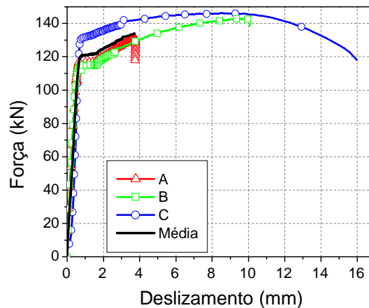
Figura 4.43 – Força vs. deslizamento da emenda 45T16EE9.5-200
