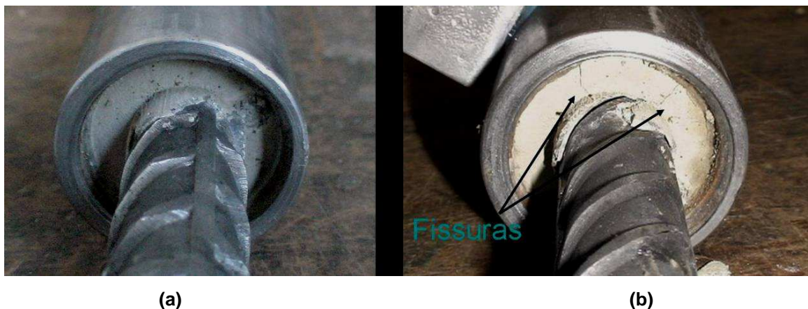
Figura 4.11 – Extremidade do transdutor 2 a) antes do ensaio e b) depois do ensaio com aparecimento de fissuras de fendilhamento
