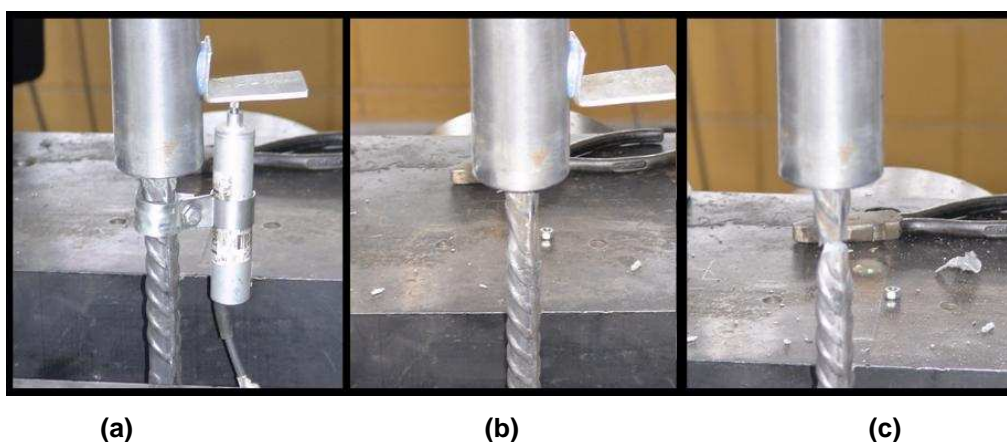
Figura 4.3 - Comportamento da barra a) Início do ensaio, b) Estrição e c) Ruína
