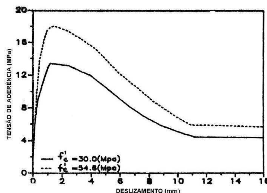
Figura 2.21 – Comportamento da aderência conforme a resistência à compressão do concreto (Eligehausen et al. , 1983, apud Soroushian et al. , 1991)
