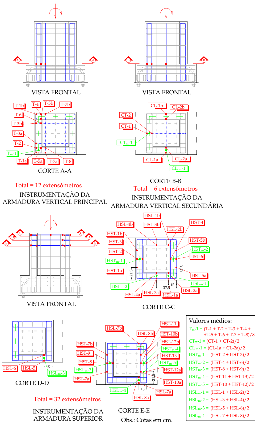
Figura 3.9: Posição dos extensômetros do Modelo IL5
