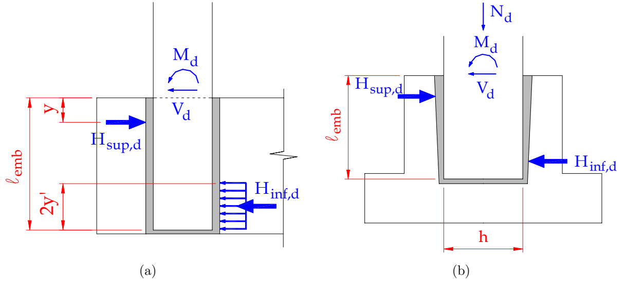
Figura 2.27: Transferência de forças: (a) AIJ; (b) DIN1045 - adaptada de CANHA(2004)
