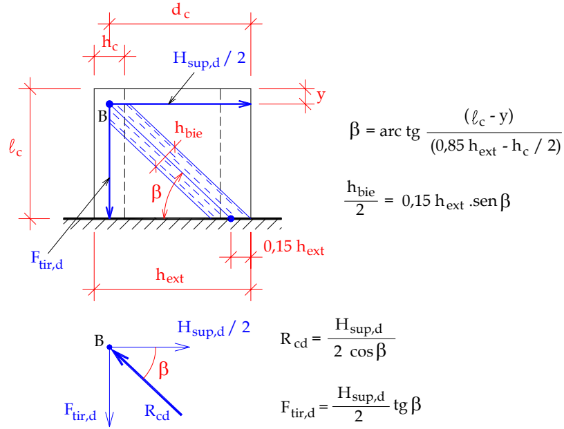
Figura 2.8: Indicações para o dimensionamento das paredes longitudinais admitindo-se comportamento de consolo curto - EL DEBS(2000) - adaptada de CANHA(2004)
