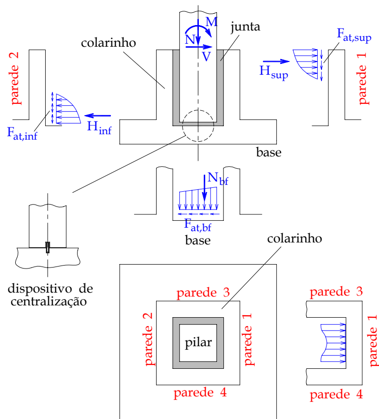
Figura 2.1: Transferência de esforços no calce de fundação com interface lisa - EL DEBS(2000) - adaptada de CANHA(2004)
