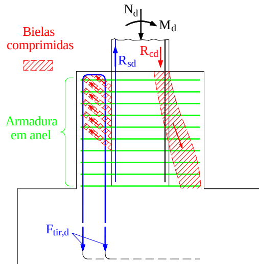
Figura 2.15: Transmissão das forças de tração e compressão no pilar sob compressão excêntrica para a fundação com interface pilar-colarinho rugosa - LEONHARDT & MÖNNIG (1977) - adaptada de CANHA(2004)
