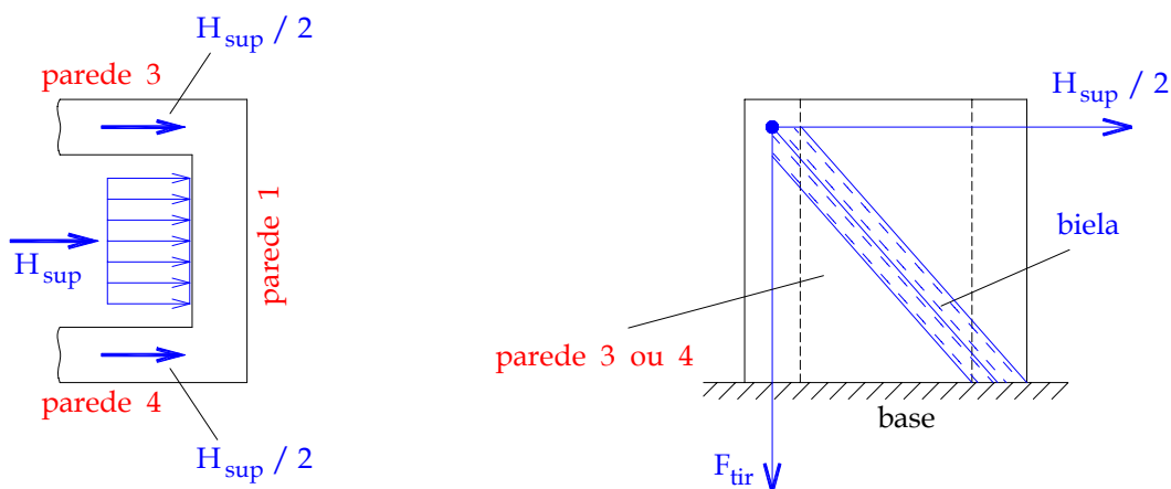
Figura 2.2: Transferência de esforços no colarinho - LEONHARDT & MÖNNIG(1977) - adaptada de CANHA(2004)
