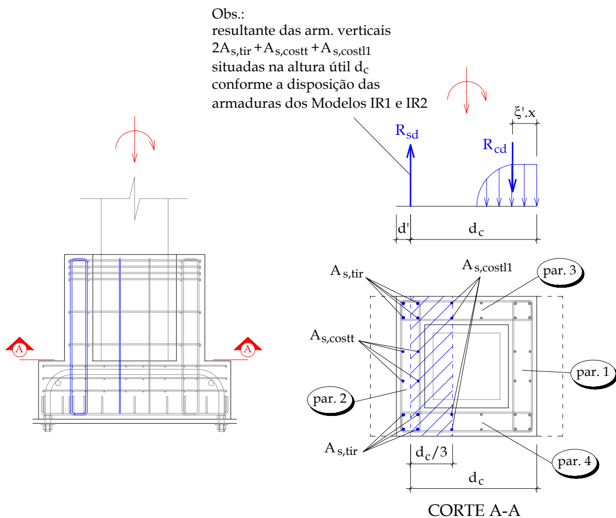
Figura 2.33: Dimensionamento das armaduras verticais para cálice com interface rugosa - CANHA(2004)
