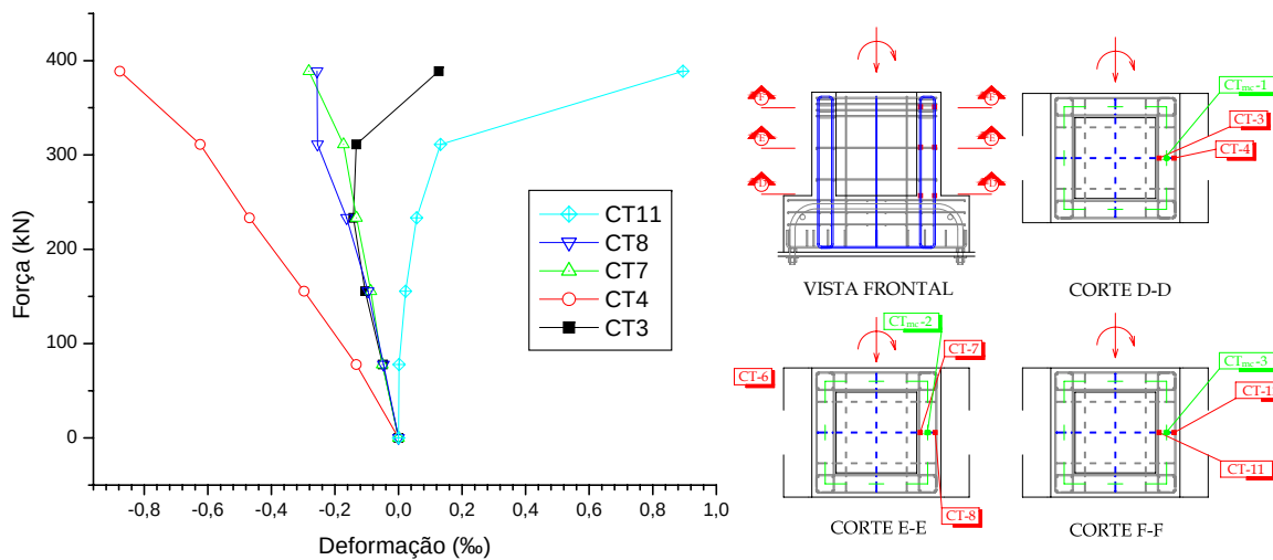
Figura 4.28: Curva força aplicada versus deformação nas armaduras verticais secundárias - Parede 1 - Modelo IR4
