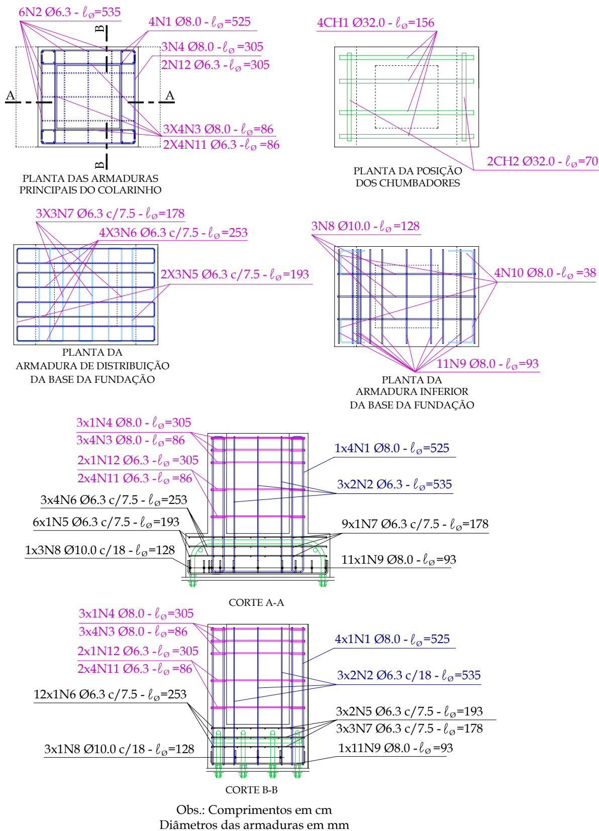
Figura 3.3: Posicionamento das armaduras do cálice de fundação para o Modelo IL5
