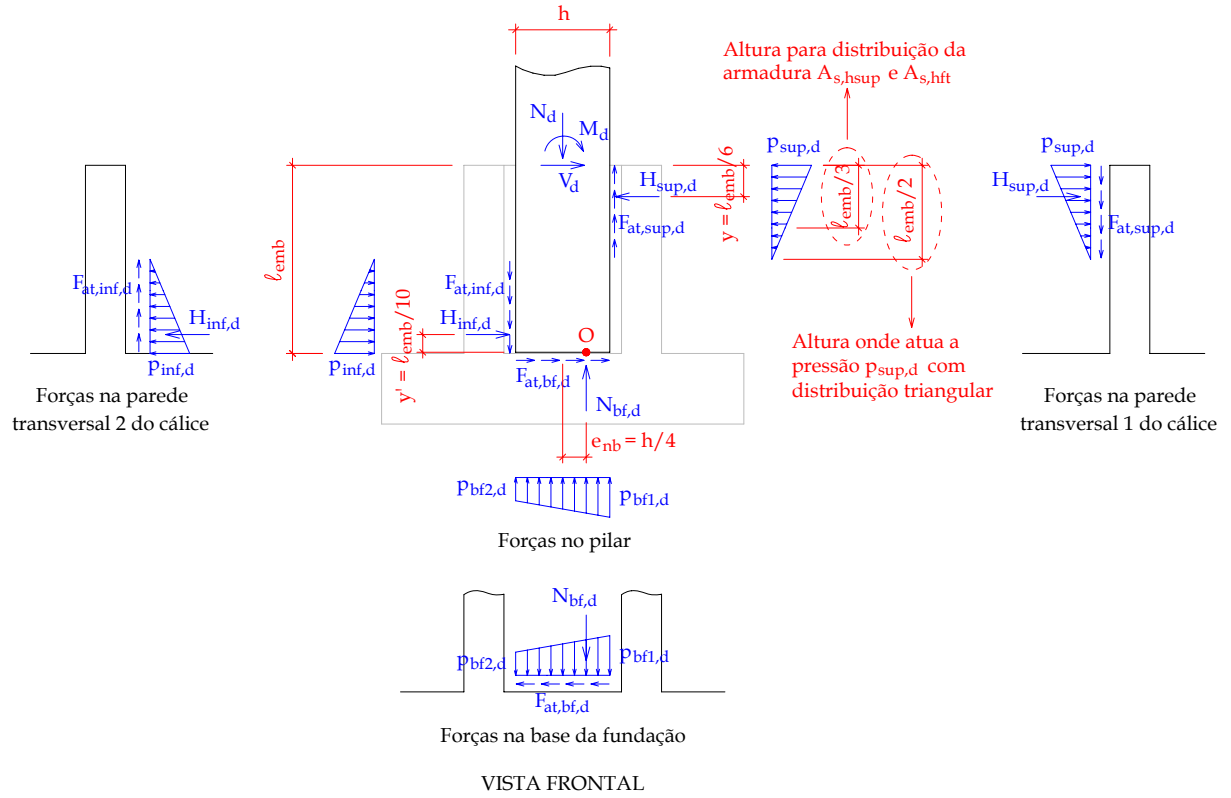
Figura 2.30: Esquema de forças atuantes do modelo de projeto proposto para cálice com interface lisa - CANHA(2004)
