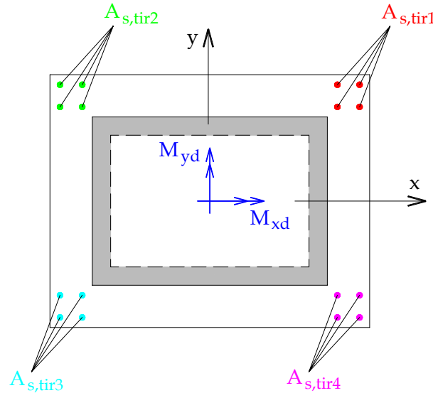
Figura 2.10: Flexão oblíqua no cálice de fundação - adaptada de CANHA(2004)
