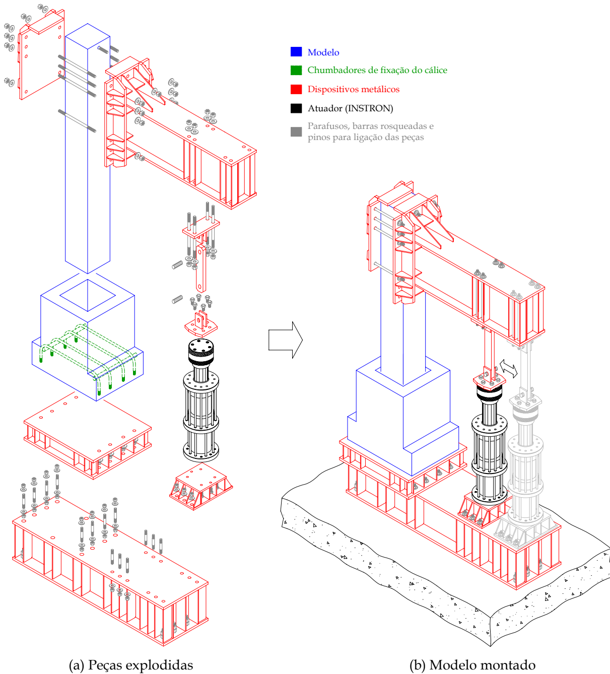
Figura 3.1: Esquema de ensaio dos modelos físicos - CANHA(2004)
