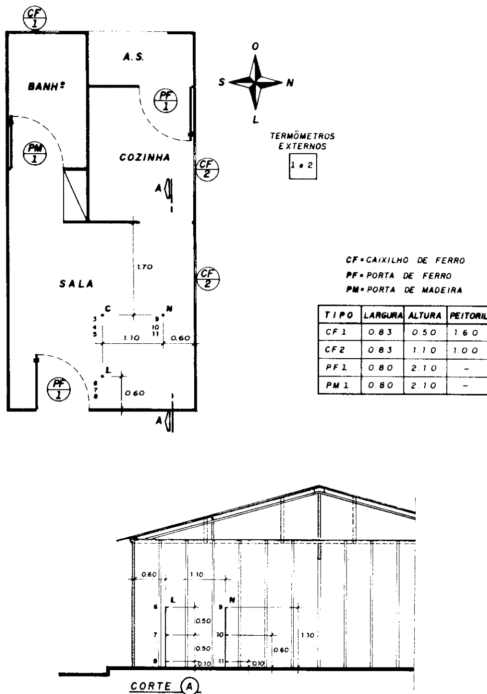
FIG. 166. ORIENTAÇÃO, CARACTERÍSTICAS DO PROTÓTIPO E POSICIONAMENTO DOS TERMÔMETROS.
