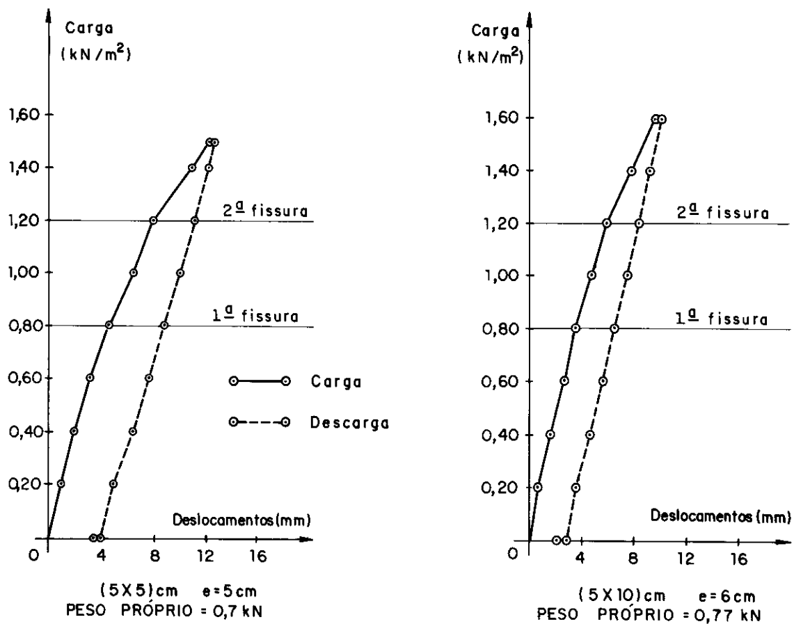
FIG. 24 - REPRESENTAÇÃO GRÁFICA DOS DESLOCAMENTOS
