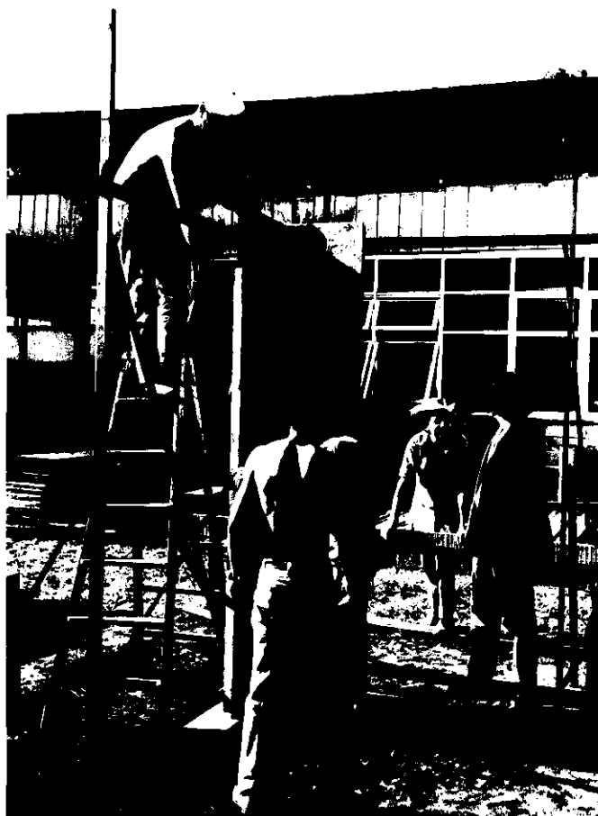
FIG. 102. INÍCIO DA MONTAGEM DAS PAREDES.
