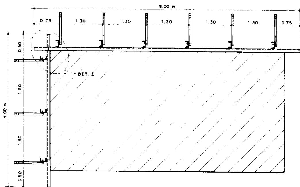
FIG. 86 - PLANTA DO ESCORAMENTO METÁLICO PARA MONTAGEM DOS PAINÉIS
