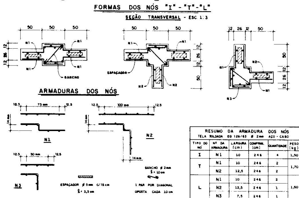
FIG. 53. FÔRMAS E ARMADURAS DOS NÓS.
