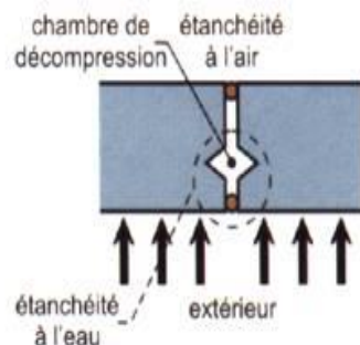
Joint vertical à deux étages
