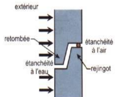
Joint horizontal à deux étages
