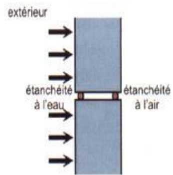
Joint horizontal à un étage
